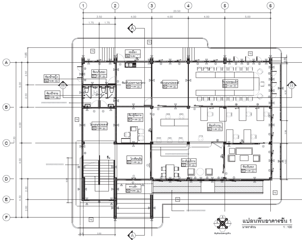
แบบแปลนอาคาร ชั้น 1
