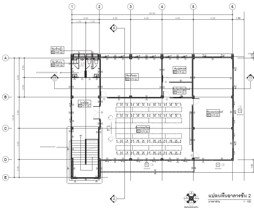
แบบแปลนอาคาร ชั้น 2
